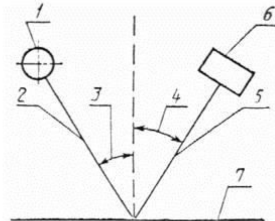
Оптическая схема методов В и Г
